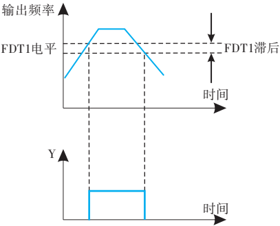
图6-25 频率水平检测示意图
