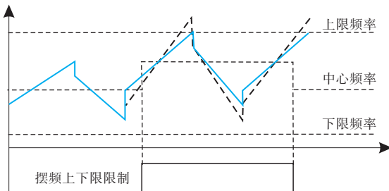
图6-23 摆频上下限限制
