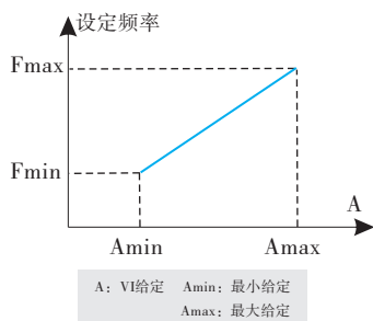
(1) 正作用特性
