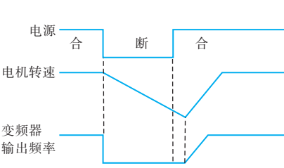
图6-09 转速跟踪再启动示意图
