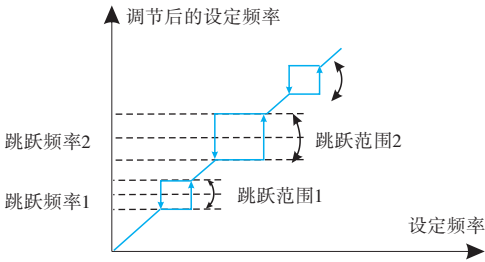
图6-15 跳跃频率及范围示意图
