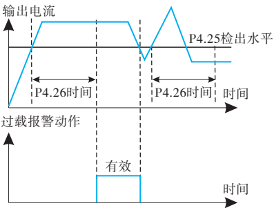
图6-27 过载报警
