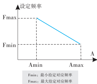
(2) 反作用特性
