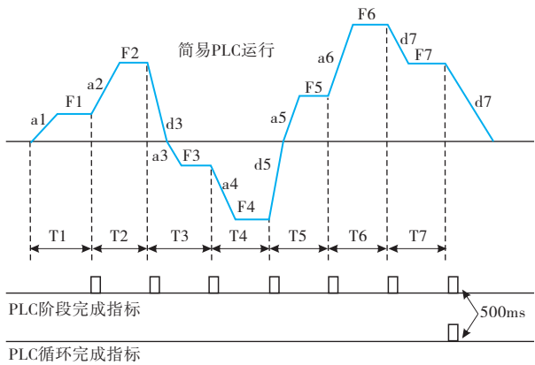
图6-33 简易PLC运行图
