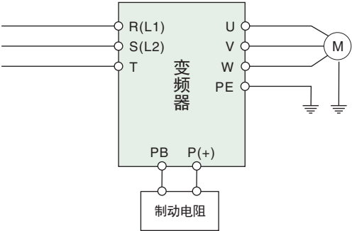
图2-9 变频器与制动组件连线图
