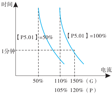
图6-25 电子热继电器保护
