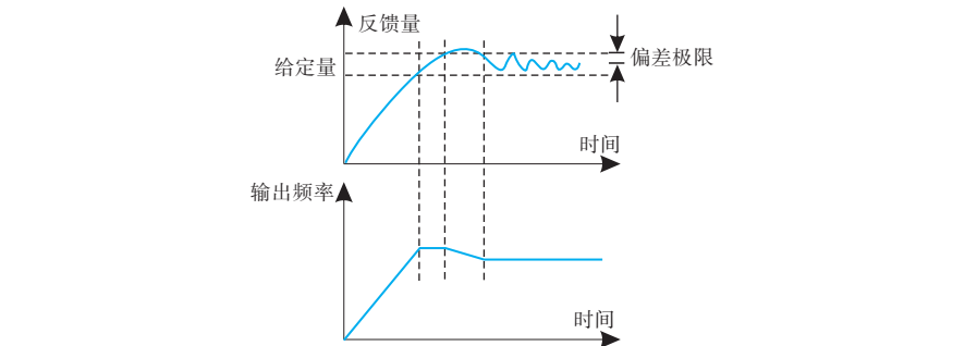
图6-31 偏差极限示意图
