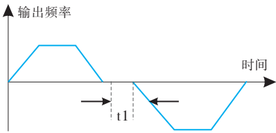
图6-01 正反转死区时间
