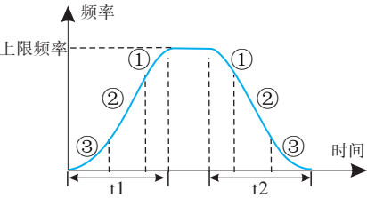
6-05 S曲线加减速
