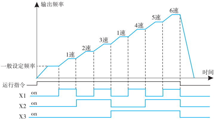
图6-16 多段速运行示意图
